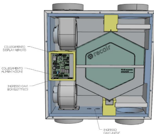
Collegamenti elettrici
