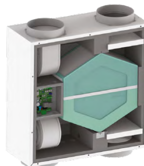
Unità di recupero 220 mc/h - es. installazione verticale
