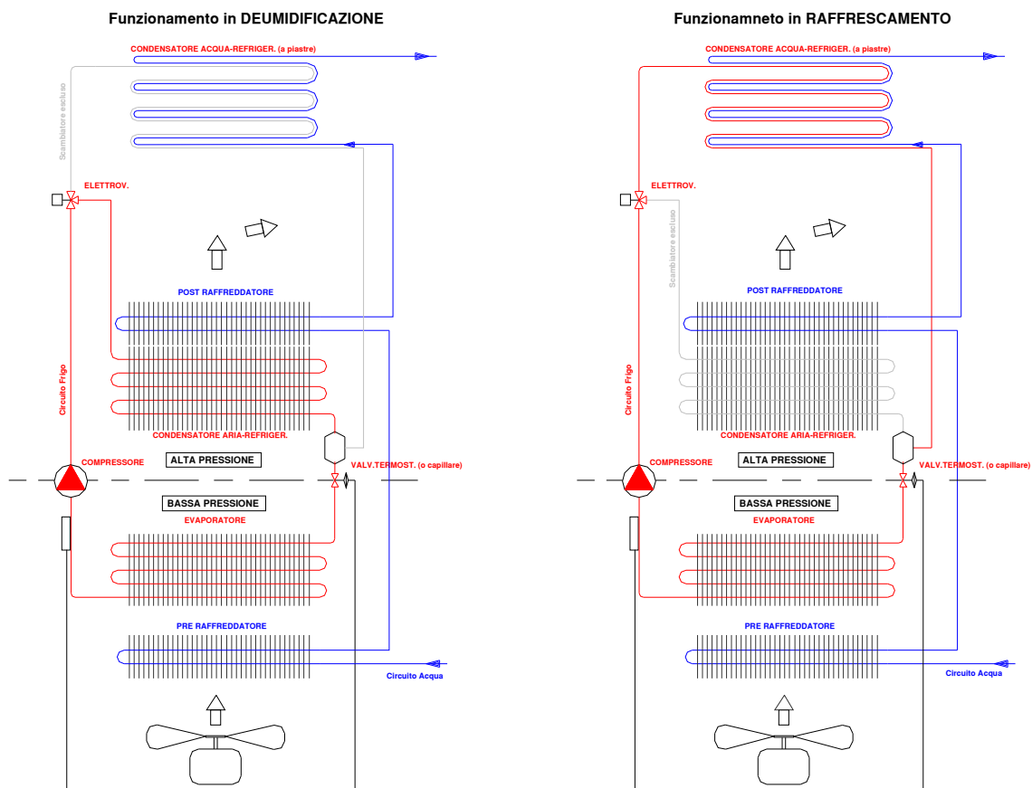
DEU - CLIMA (Brev. N° VI2005A000055) Schema funzionale (rappresenta solo una raffigurazione del concetto)
