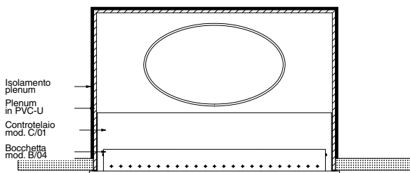
SEZIONE VISTA LATO LUNGO (con bocchetta, da ordinare a parte)
