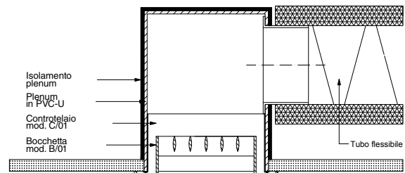
SEZIONE VISTA LATO CORTO (con bocchetta, da ordinare a parte)
