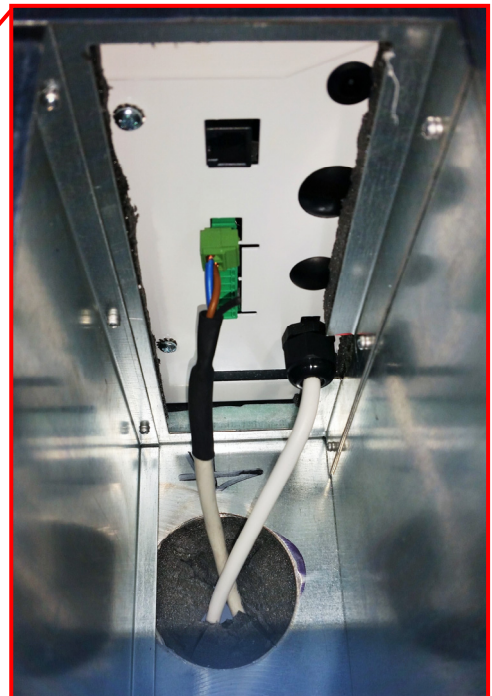
PARTICOLARE COLLEGAMENTI ELETTRICI DI ALIMENTAZIONE E PANNELLO AIRCONTROL
